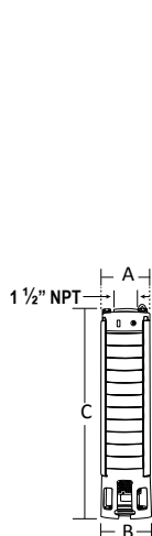
Acoplamiento NEMA 4"
