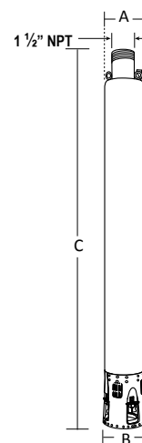
Acoplamiento NEMA 6"
