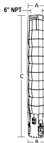
Acoplamiento NEMA 8" Fig. 2
