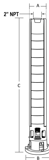
Acoplamiento NEMA 6"
