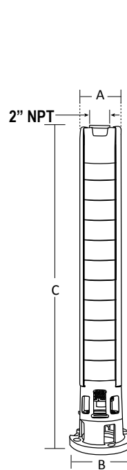
Acoplamiento NEMA 6"
