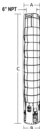
Acoplamiento NEMA 8" Fig. 1
