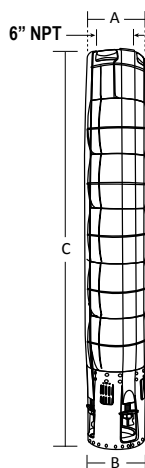
Acoplamiento NEMA 8"
