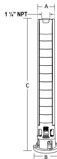
Acoplamiento NEMA 6"
