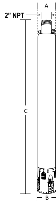
Acoplamiento NEMA 6"
