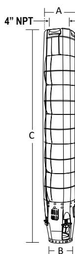
Acoplamiento NEMA 4" Fig. 1
